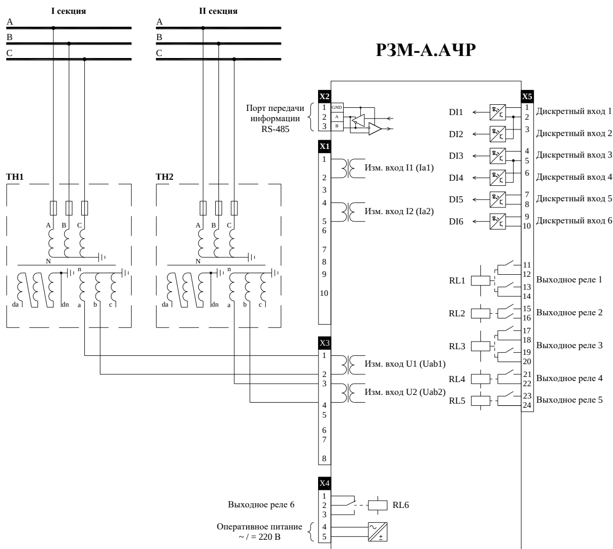
Рисунок 2. Схема подключения РЗМ-А.АЧР с модулем входов/выходов - 6DI-6RL.
