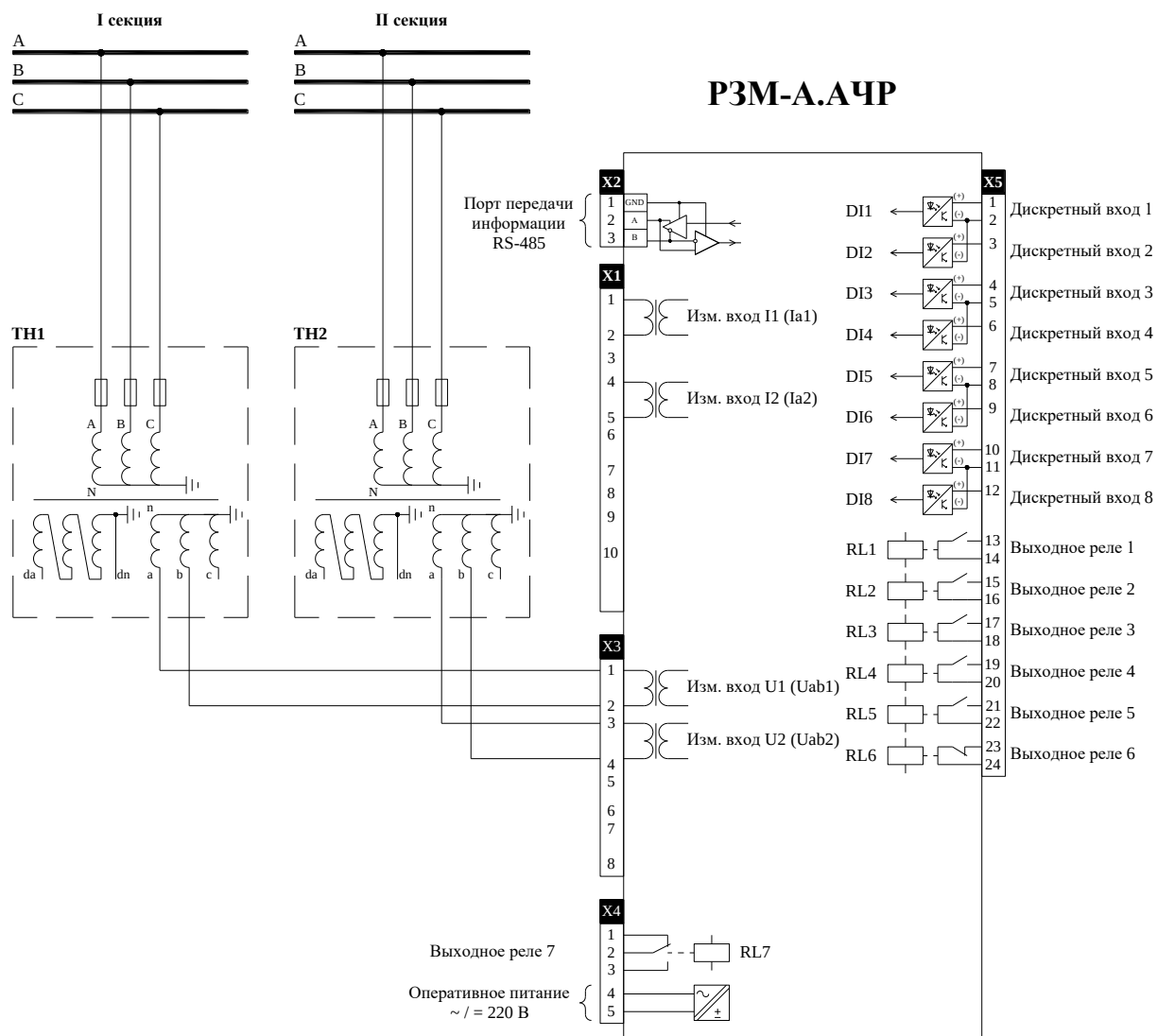
Рисунок 3. Схема подключения РЗМ-А.АЧР с модулем входов/выходов - 8DI-7RL.
