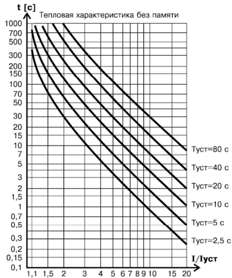
6. Тепловая характеристика без памяти.
