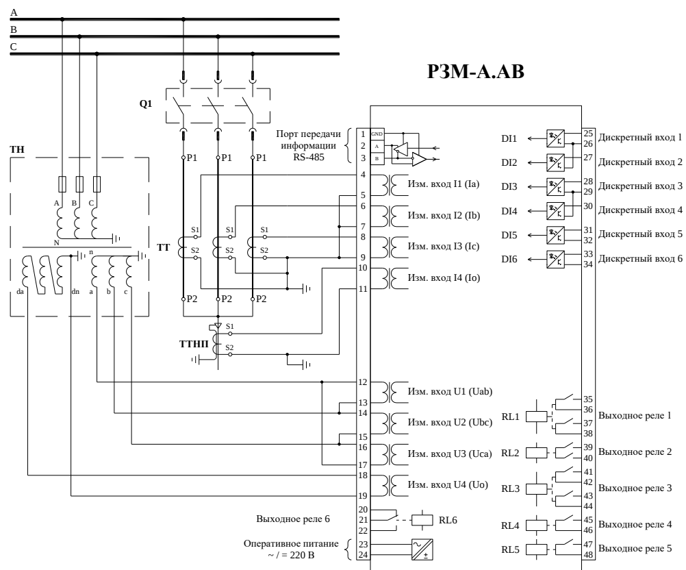
Рисунок 1. Схема подключения РЗМ-А.АВ с модулем входов/выходов - 6DI-6RL и зажимами WAGO.
