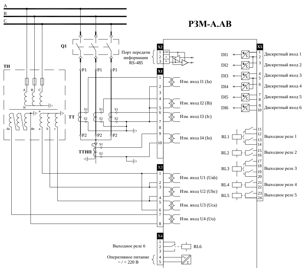
Рисунок 2. Схема подключения РЗМ-А.АВ с модулем входов/выходов - 6DI-6RL и винтовыми зажимами.
