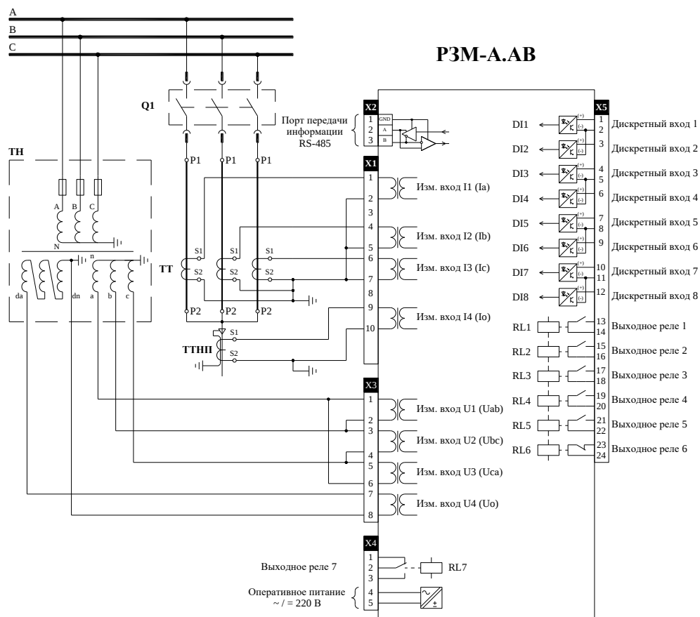
Рисунок 3. Схема подключения РЗМ-А.АВ с модулем входов/выходов - 8DI-7RL
