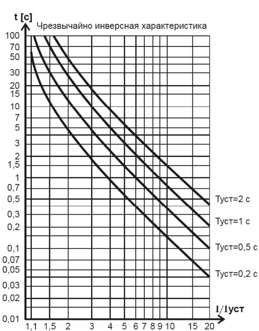
3. Чрезвычайно инверсная характеристика по МЭК 255-4.
