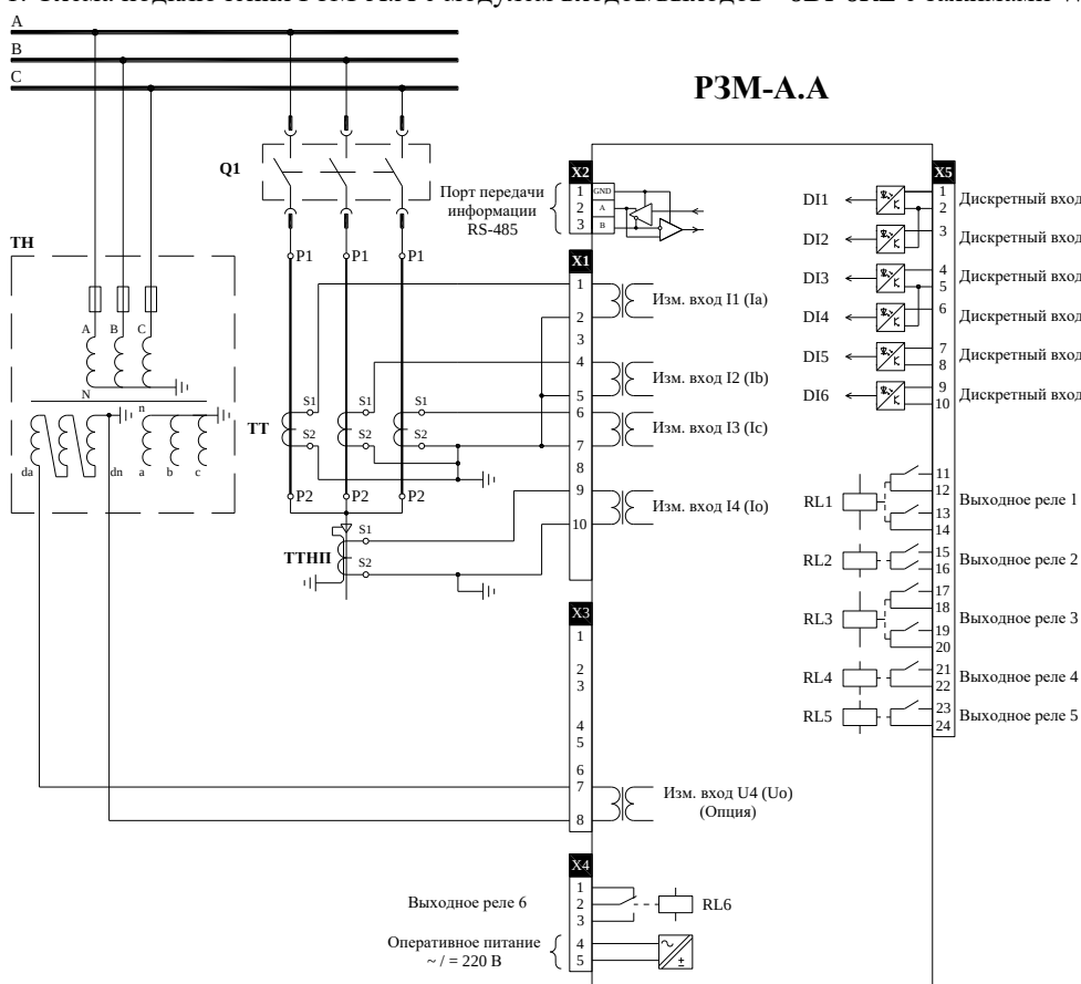
Рисунок 1. Схема подключения РЗМ-А.А с модулем входов/выходов - 6DI-6RL с зажимами WAGO.
