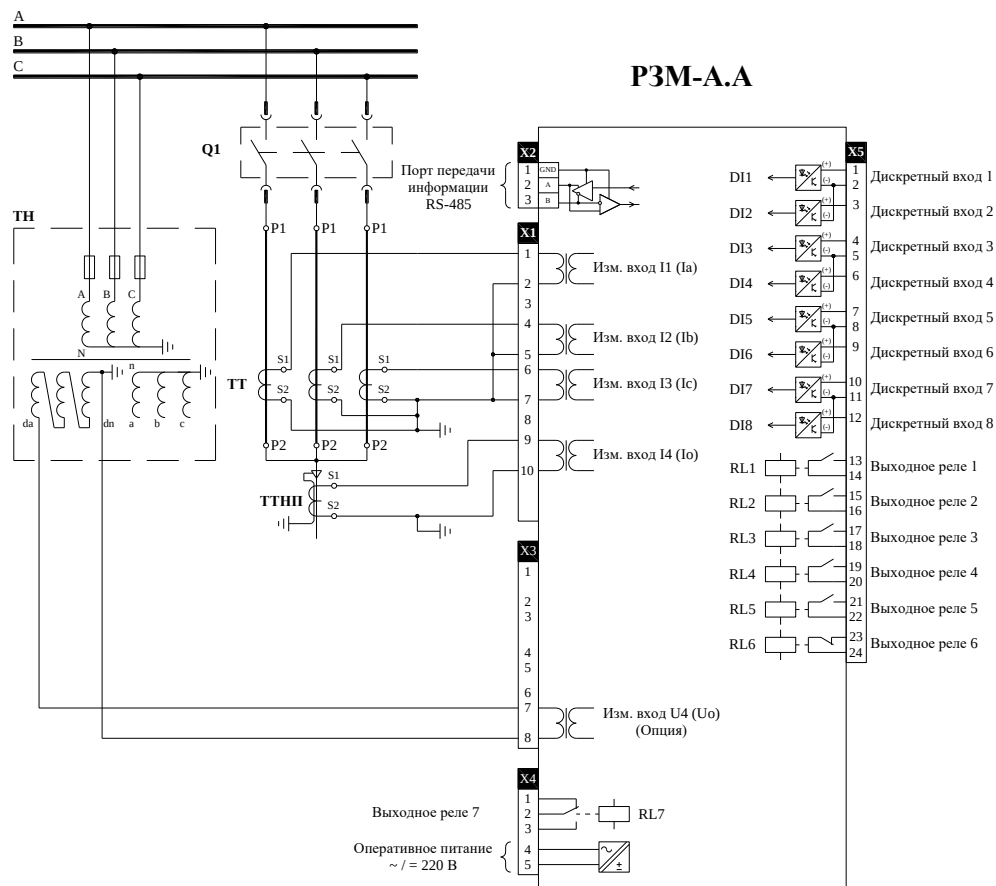
Рисунок 3. Схема подключения РЗМ-А.А с модулем входов/выходов - 8DI-7RL.
