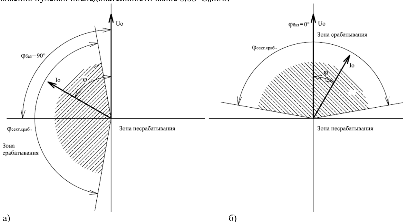
Рисунок 1. – диаграмма определения направления и зоны срабатывания НЗНЗ
