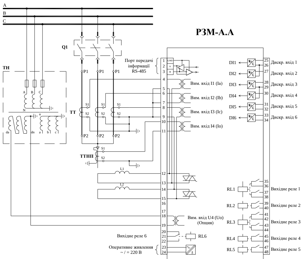
Рисунок 4. Схема подключения РЗМ-А.А с модулем входов/выходов - 6DI-6RL с зажимами WAGO и выходами дешунтирования электромагнитов отключения.
