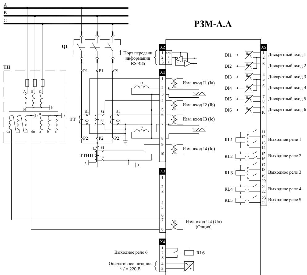
Рисунок 5. Схема подключения РЗМ-А.А с модулем входов/выходов 6DI-6RL с винтовыми зажимами и выходами дешунтирования электромагнитов отключения.
