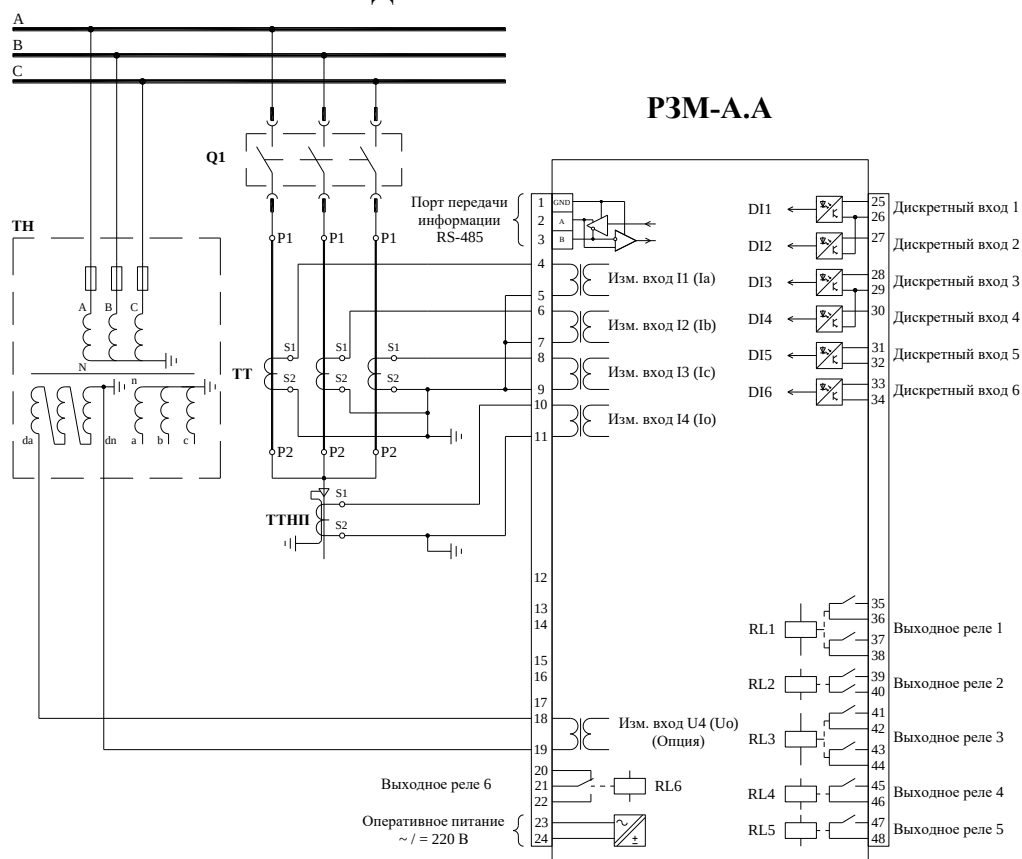
Рисунок 1. Схема подключения РЗМ-А.А с модулем входов/выходов - 6DI-6RL с зажимами WAGO.
