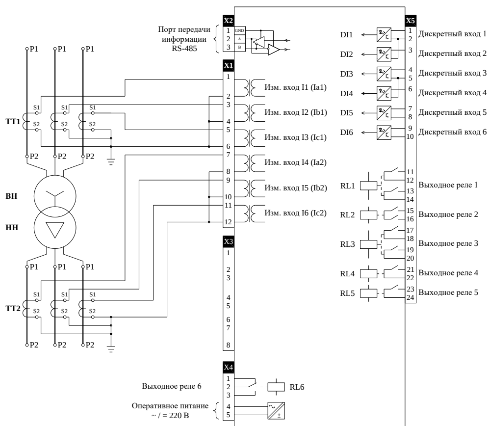
Рисунок 2. Схема подключения РЗМ-А.Т2 с модулем входов/выходов - 6DI-6RL и винтовыми зажимами.
