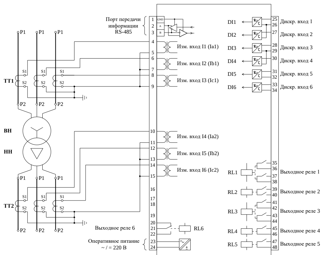
Рисунок 1. Схема подключения РЗМ-А.Т2 с модулем входов/выходов - 6DI-6RL с зажимами WAGO
