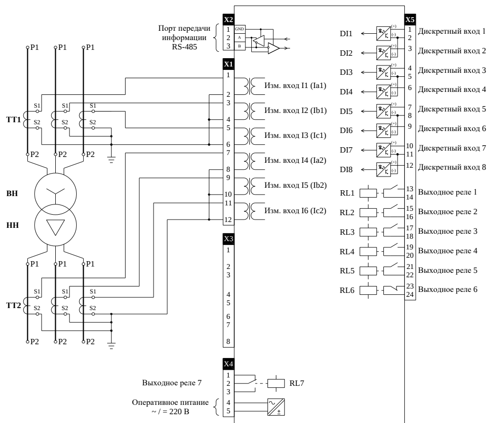
Рисунок 3. Схема подключения РЗМ-А.Т2 с модулем входов/выходов - 8DI-7RL.
