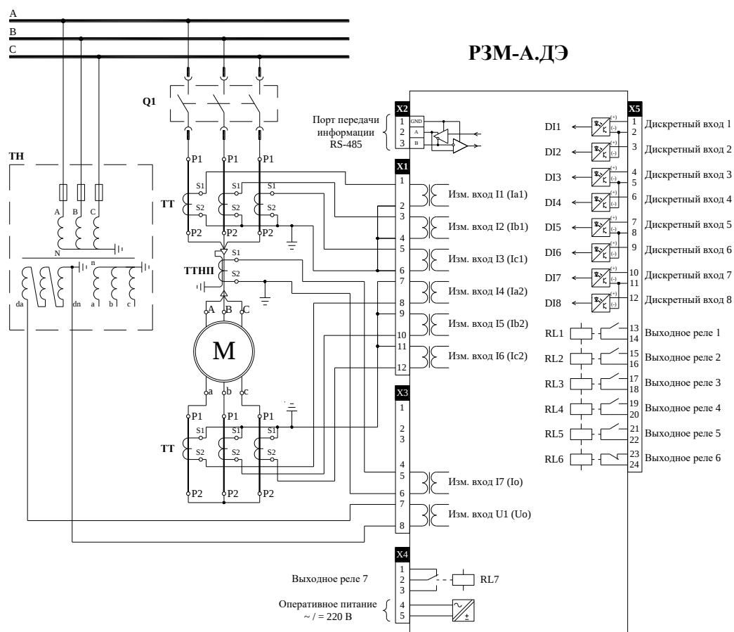
Рисунок 3. Схема подключения РЗМ-А.ДЭ с модулем входов/выходов - 8DI-7RL.
