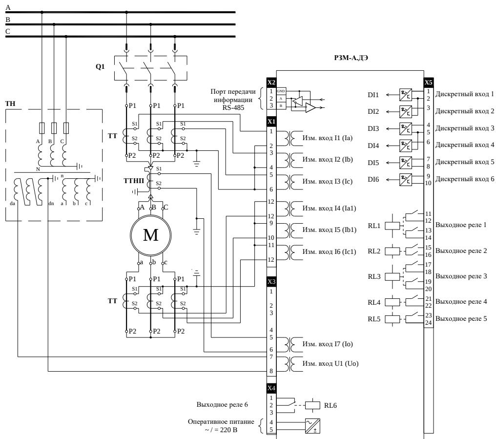
Рисунок 1. Схема подключения РЗМ-А.ДЭ с модулем входов/выходов - 6DI-6RL и зажимами WAGO
