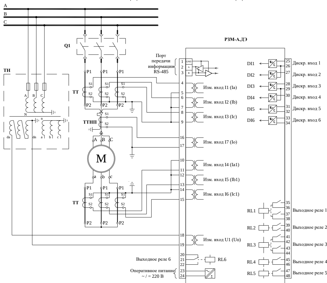
Рисунок 1. Схема подключения РЗМ-А.ДЭ с модулем входов/выходов - 6DI-6RL и зажимами WAGO
